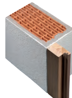
Blendrahmen BM 43/65* in der Laibung montiert (beliebige Position)
