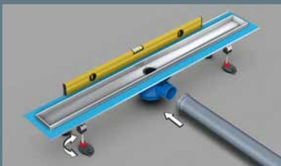
Шаг 1 - Сборка дренажного канала, выравнивание канала по горизонтали с помощью опор, подключение к канализации
